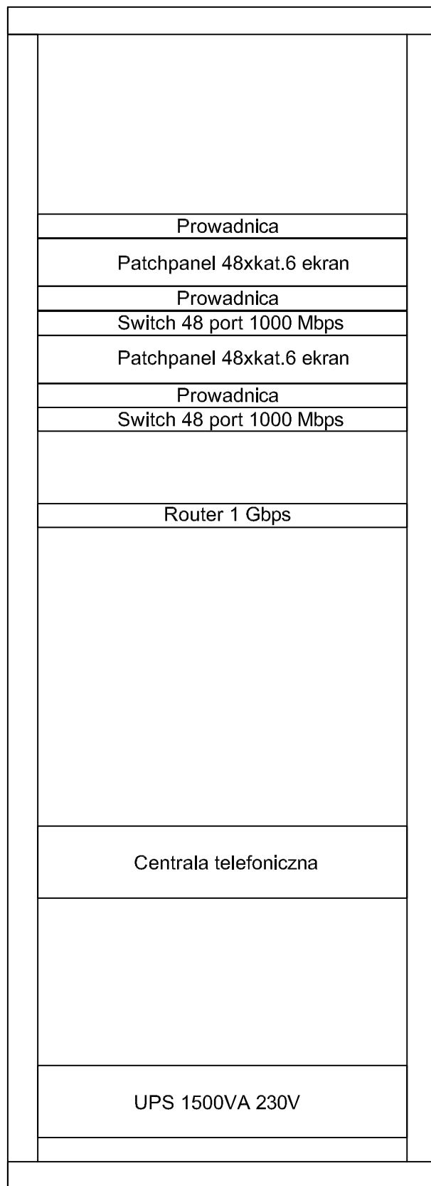
Szafa stojąca 19" 47U 800/800/2195mm, drzwi przeszkłone
